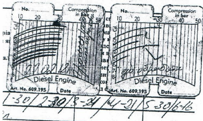
Рис.1. Диаграммы компрессии двигателя автомобиля MAN 14.84, Гос. № АР 5987 ВС
